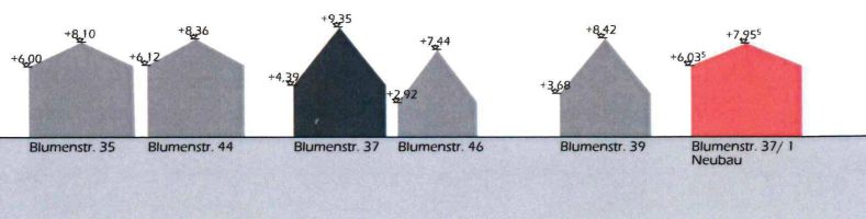
Höhenabwicklung best. Gebäude Blumenstraße M 1:500
